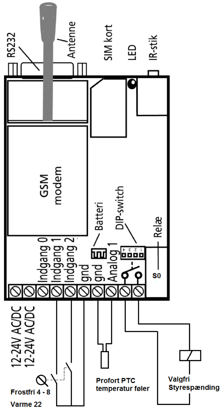
Fig. 1 Profort enhed multiGuard Micro/Duplex 312
